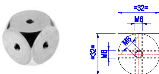
6070-008-003 ( 601160 ) BOXCORNERKNOB M6
